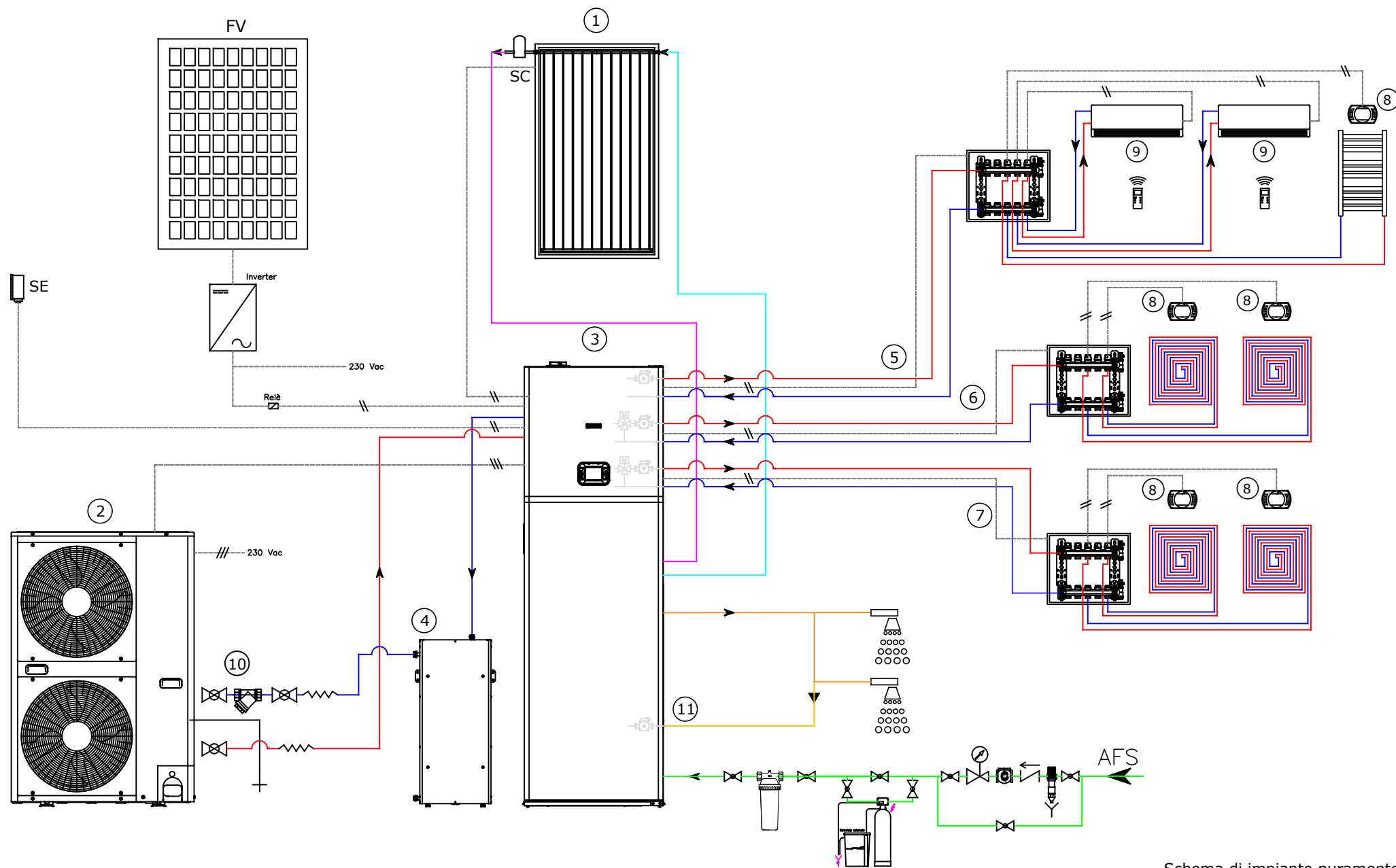
Schema di impianto puramente indicativo
